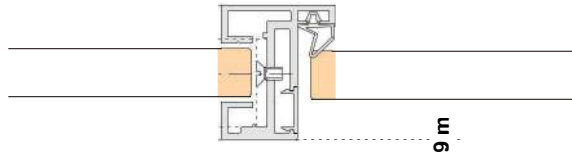
ATC 45 Freestanding door frame profile
